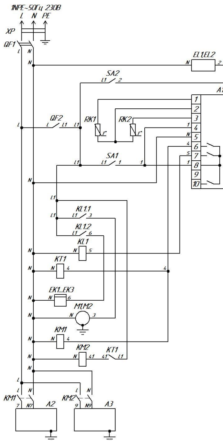
Схема электрическая принципиальная
